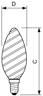
filament 2.5W-25W 250lm NAD 2200K E14ND
